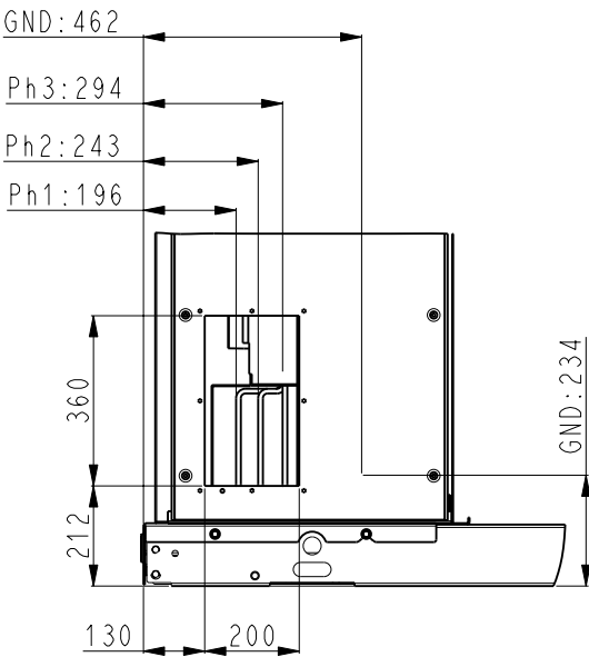
VUE / VIEW B
