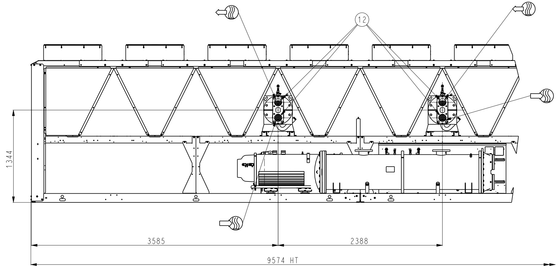
VUE F ECHELLE 1:32
