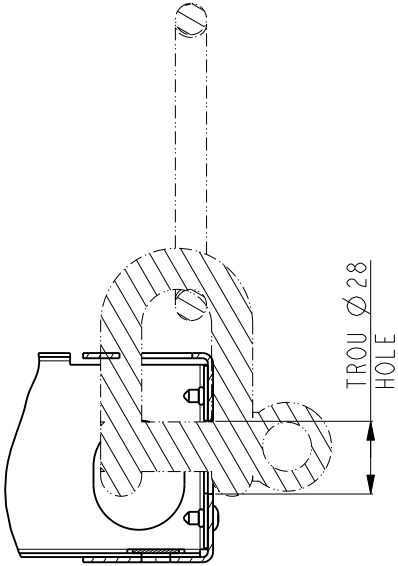
COUPE / SECTION B-B Echelle 11:32
