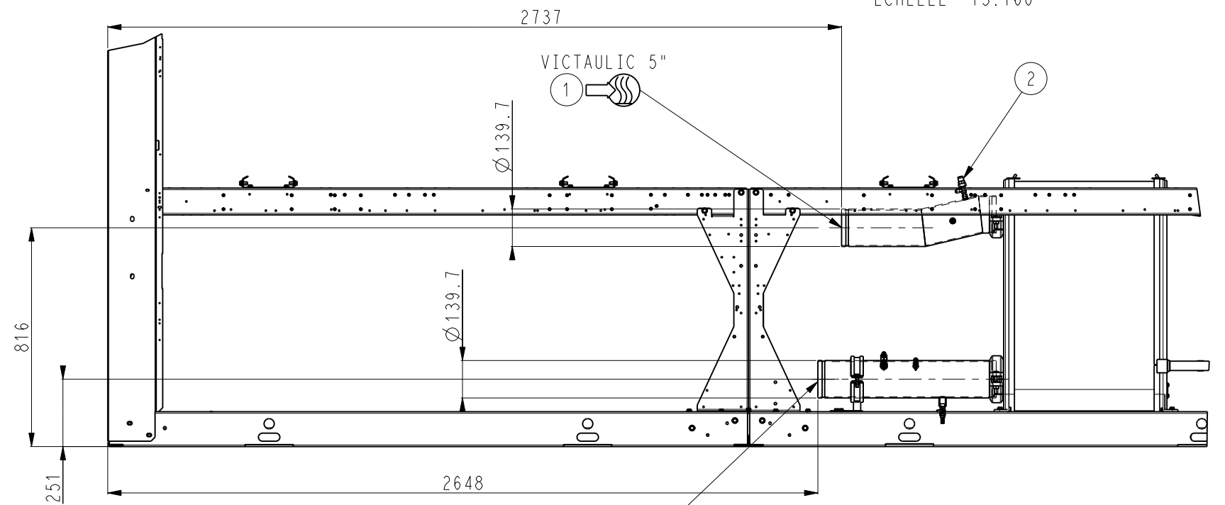
1 VICTAULIC 5"
