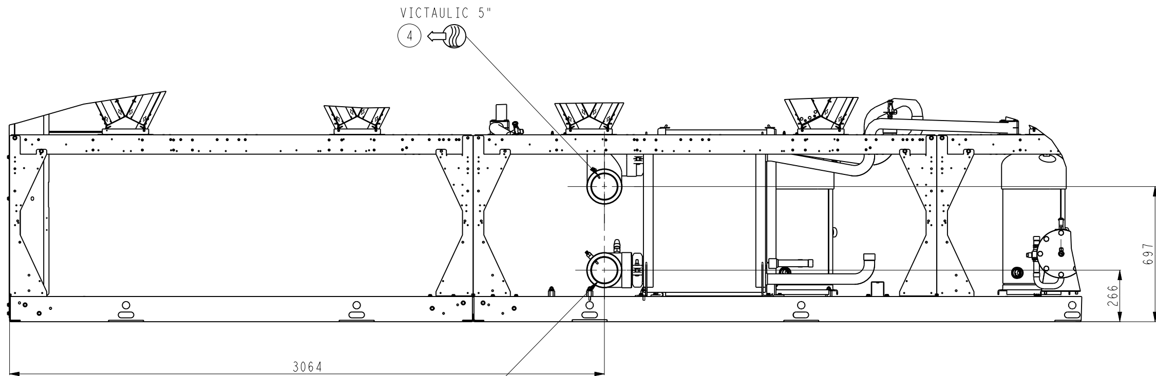
4 VICTAULIC 5"
