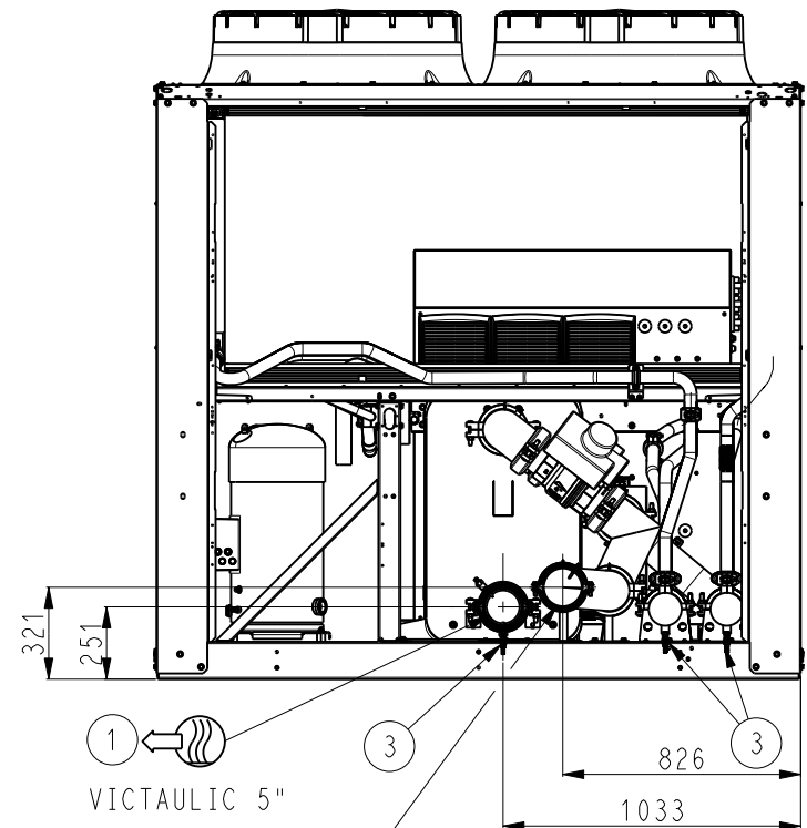
1 VICTAULIC 5"
