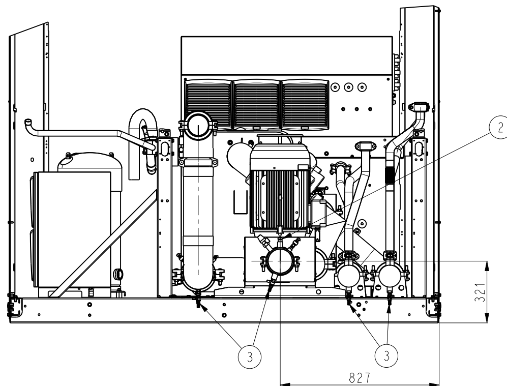
VUE H VIEW ECHELLE 1:20
