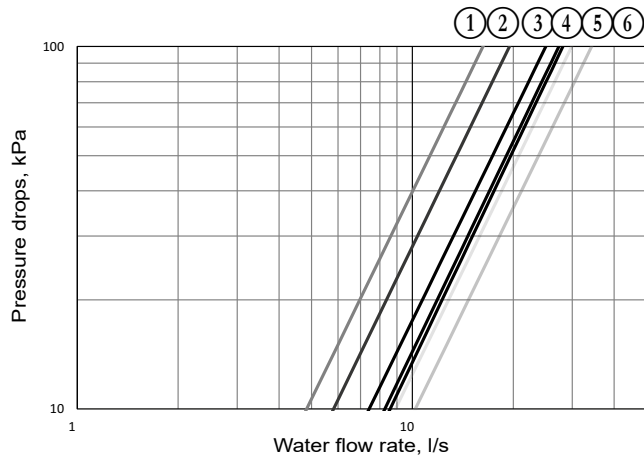
Sizes 170R - 550R
