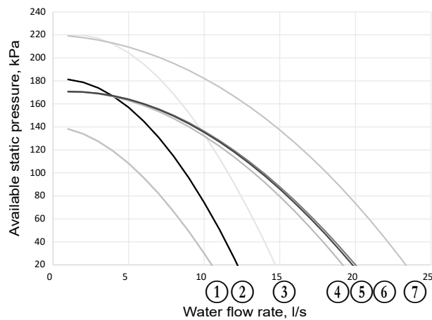
Sizes 170R - 410R
