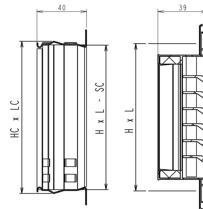
COUPE / SECTOIN A-A
