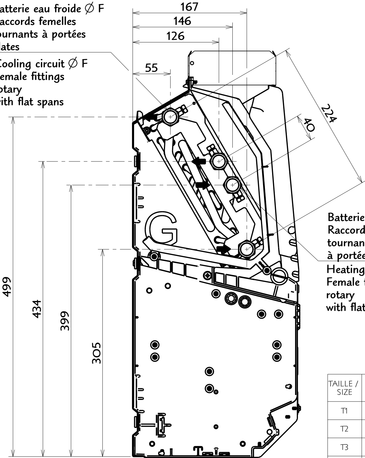
BATTERIE 4T (PRISES A GAUCHE) / COIL 4T (LEFT HAND CONFIGURATION)
