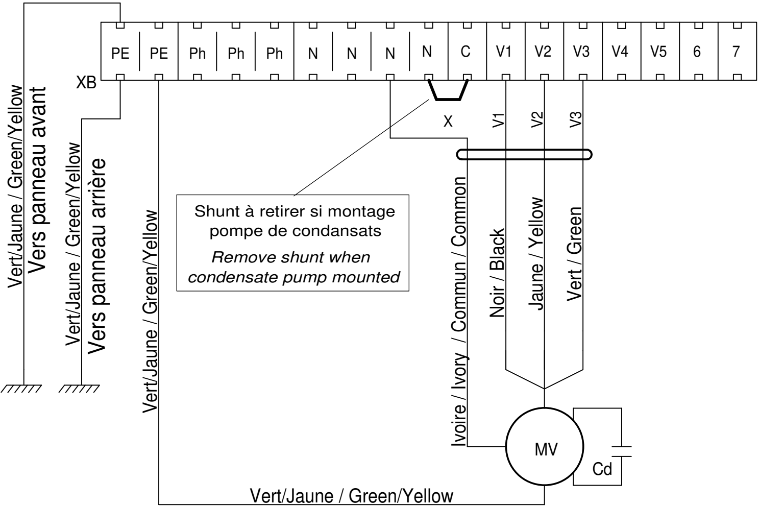
Moteur 3 vitesses (Modèles 42NX235 ou 42NX336) 3 speeds motor (42NX235 ou 42NX336 Models)
