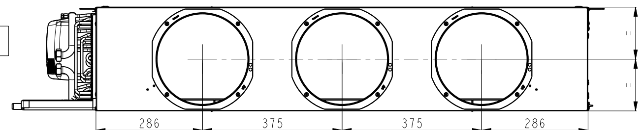
42NX T5 VUES FACE AU SOUFFLAGE FRONT VIEW AIR SUPPLY
