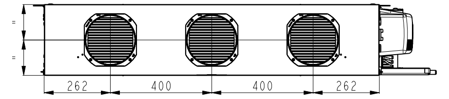
42NX T5 VUES ARRIERE A LA REPRISE BACK VIEW AIR RETURN
