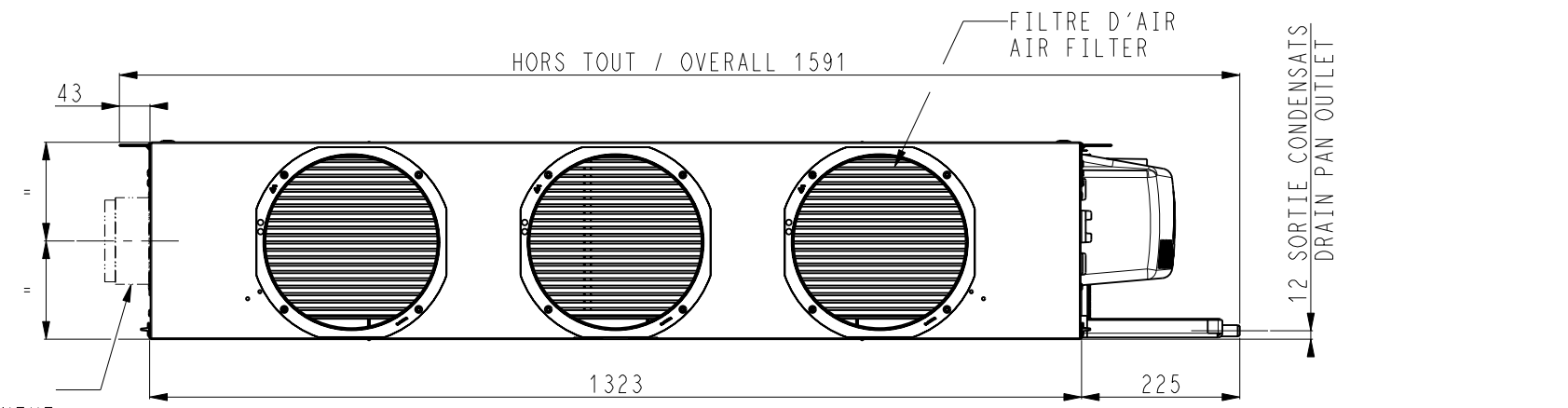
42NX T5 VUE FACE AU SOUFFLAGE FRONT VIEW AIR SUPPLY
