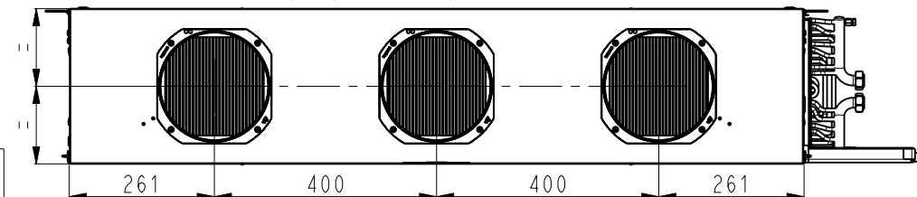
42NX T5 VUES ARRIERE A LA REPRISE BACK VIEW AIR RETURN
