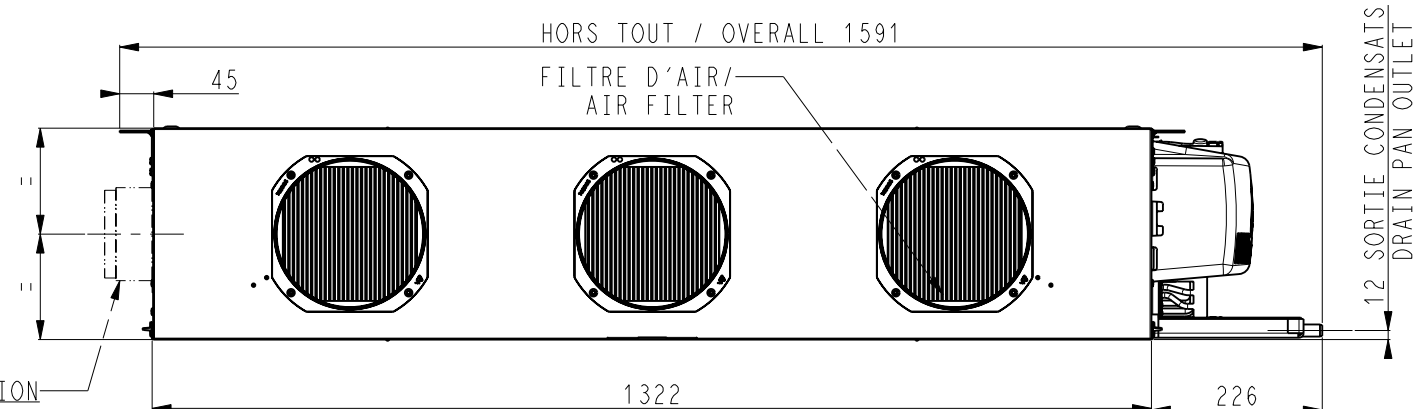
VUES FACE AU SOUFFLAGE FRONT VIEW AIR SUPPLY
